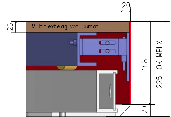
Detaildarstellung mit optionaler Randblende
